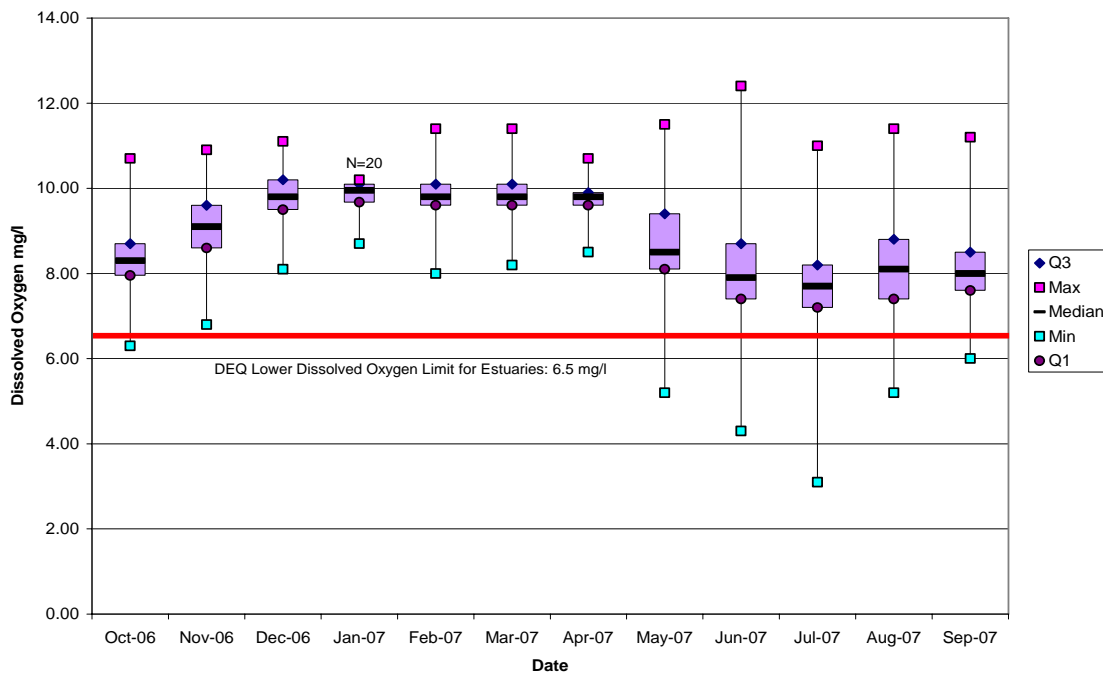
Boxplot8
